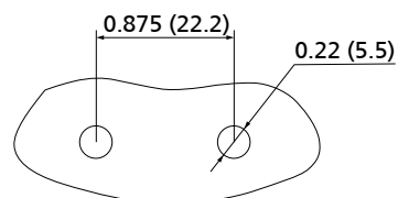
底部安装固定开孔
