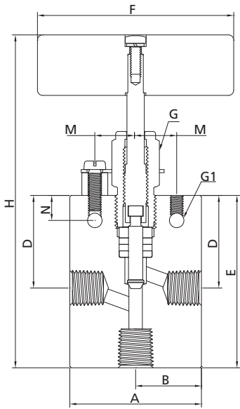
3通/2进
