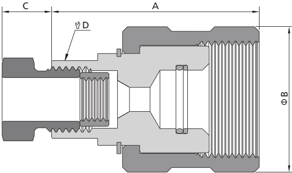
母接头
