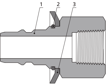
公接头
