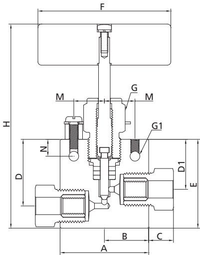
直通型
