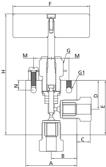
角型
