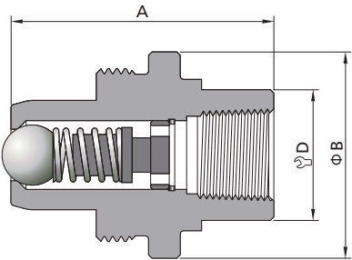
公接头
