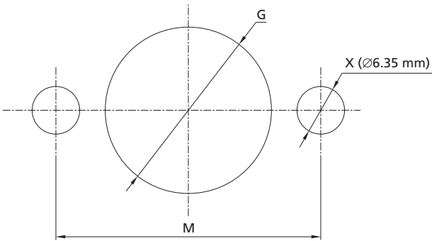
面板安装示意图
