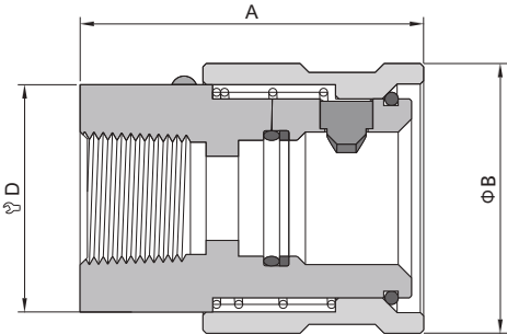
母接头
