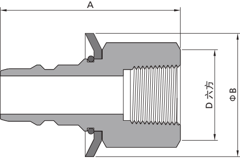
公接头
