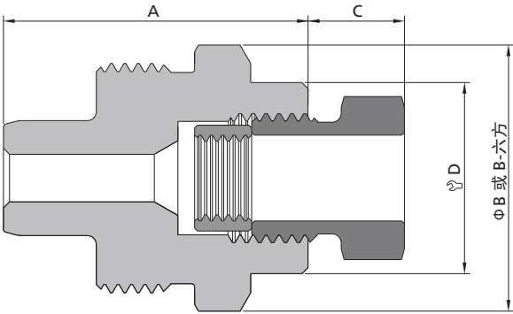
公接头
