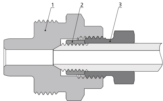
公接头
