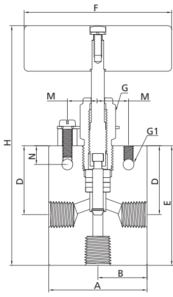
3通/1进
