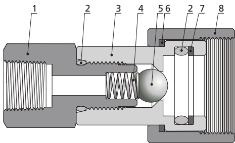
母接头
